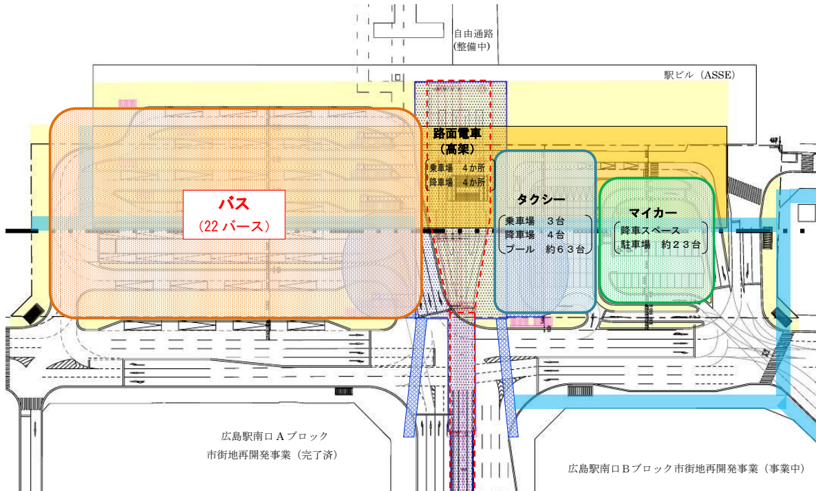
図-63 広島駅南口広場再整備の計画平面図（案）
